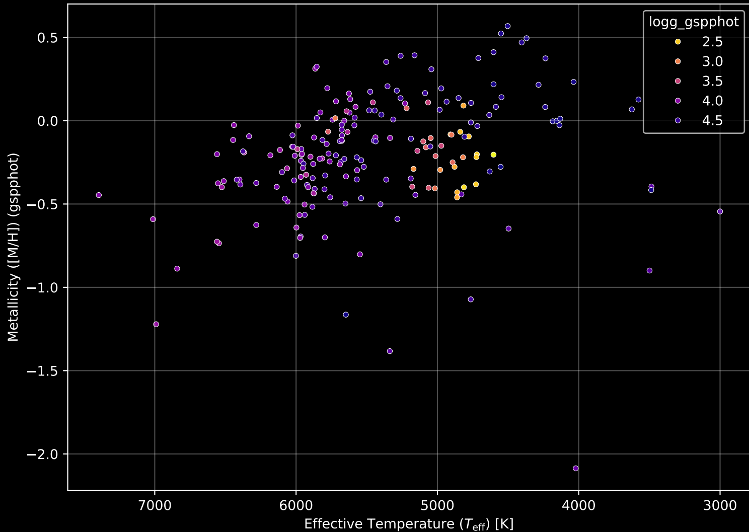
APOGEE DR17 Field: [175+58_MGA] Stellar Population Parameters (n= 200)
